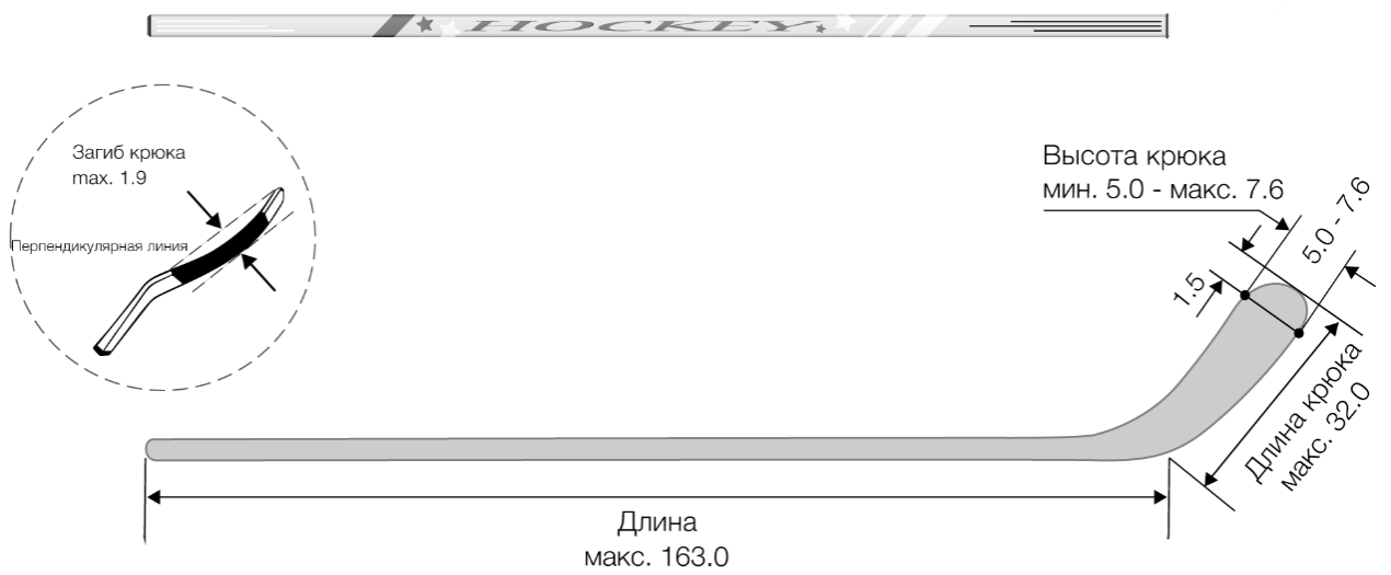
Рисунок 26. Клюшка игрока
