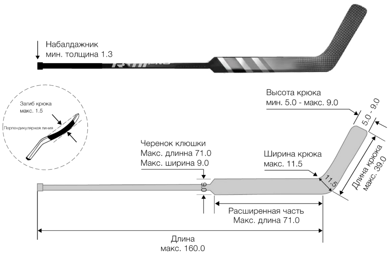
Рисунок 27. Клюшка вратаря
